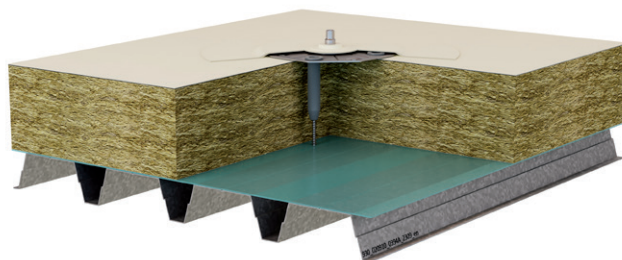
Festebrakett festet med SFS ISOTAK skruer og hylser.
