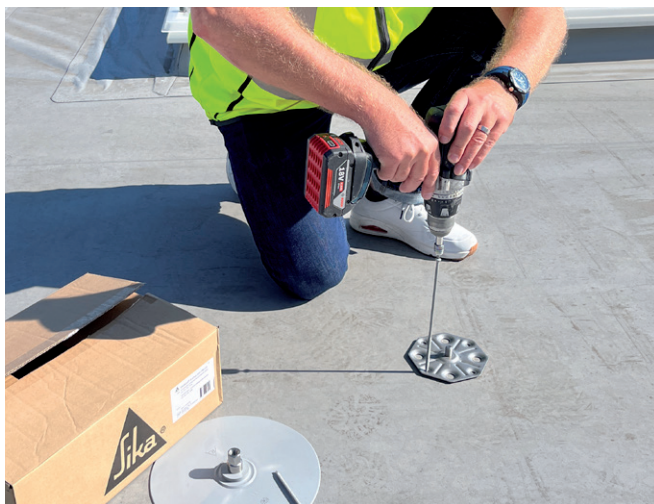
Brakett festes med SFS ISOTAK skruer og hylser.
