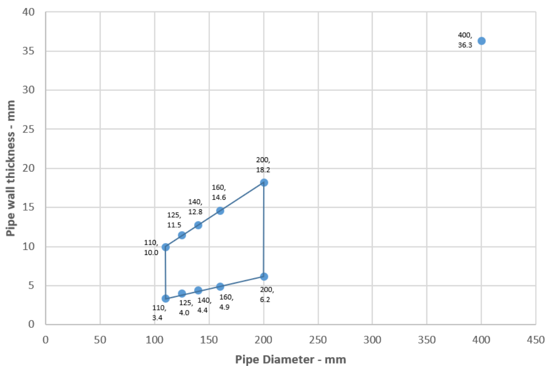
PE Pipes
